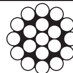
19 fios 1+6/12
