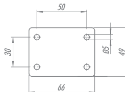
Placa ESM *Opcional para linha 158/210
