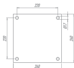
YPEX 64 a 124 • DOLLY GDE/GDERX
