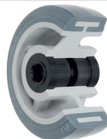
BUCHA DE NYLON COM MANGA DE EIXO
