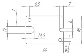
Placa GLP/GLDP *Opcional para linha 158/210
