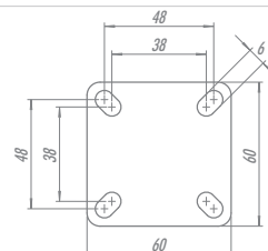
Placa P60 *Opcional para linha 158/210
