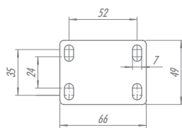
Placa GL/GLD *Opcional para linha 158/210
