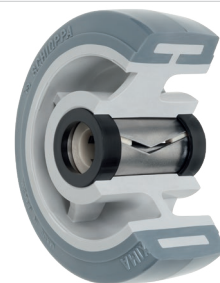
ROLAMENTO DE ROLETES COM CAPA
