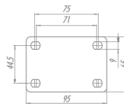
Placa LA *Opcional para linha 158/210/212
